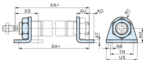
脚架安装件 HBN
