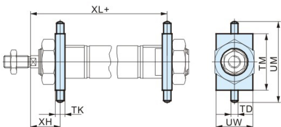
耳轴安装件 WBN
