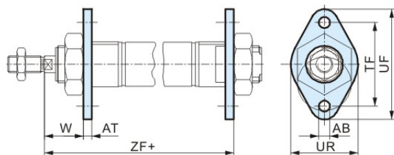
法兰安装件 FBN
