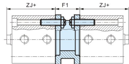
多位置组建DPNC
