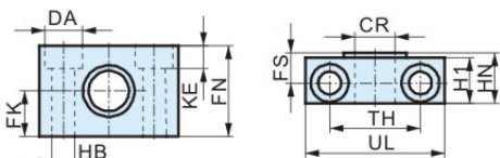
耳轴支座LNZG
