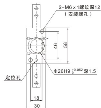
磁性开关安装槽位置
