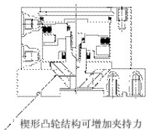
楔形凸轮结构可增加夹持力
