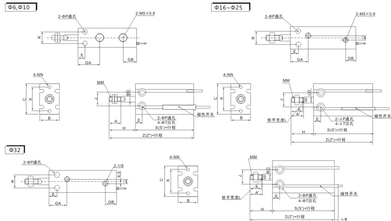
共同尺寸表
