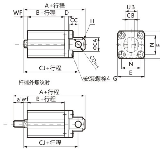
双耳环(CB)不带开关 SSD2-12~25-CB
