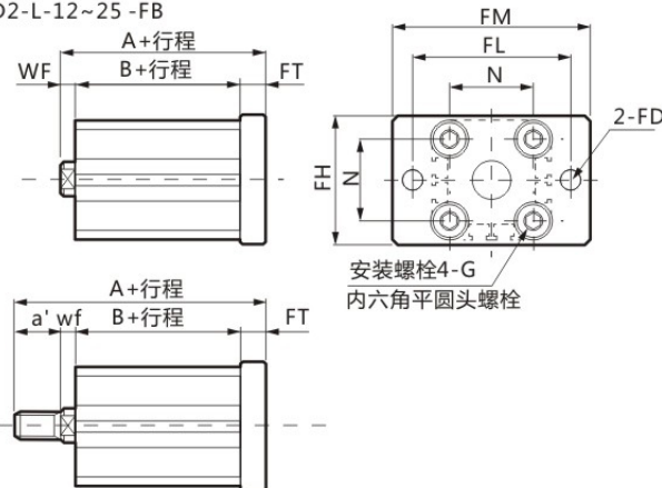
后端法兰(FB)带开关 SSD2-L-12~25-FB
