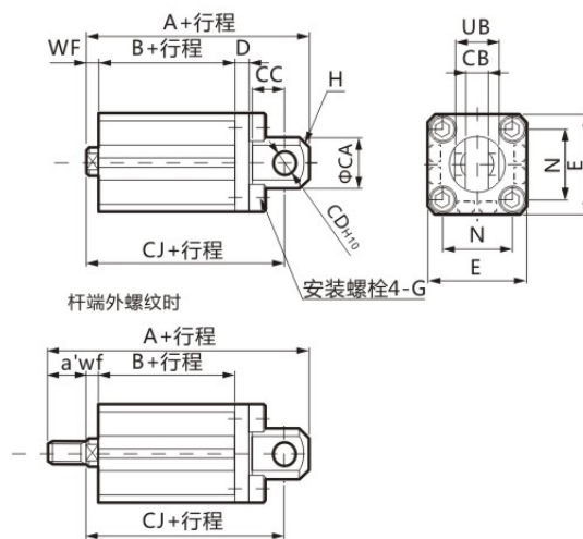
双耳环(CB)带开关 SSD2-L-12~25-CB
