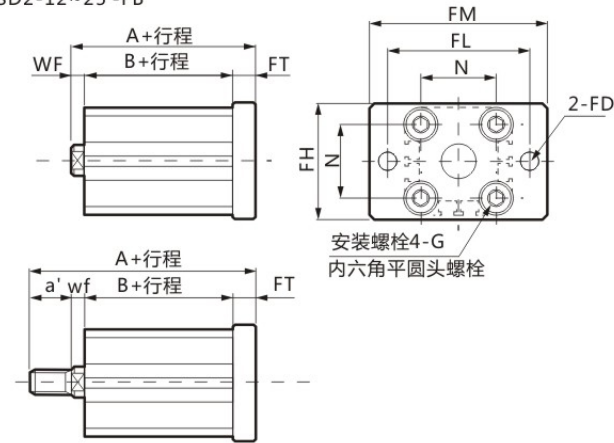
后端法兰(FB)不带开关 SSD2-12~25-FB
