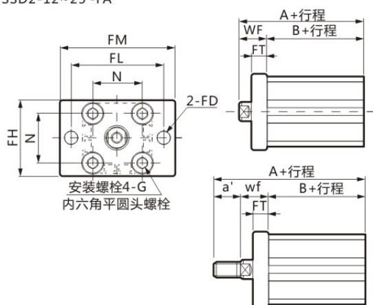
前端法兰(FA)不带开关 SSD2-12~25-FA
