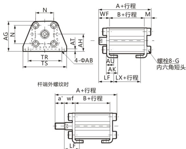
轴向脚座(LB)不带开关 SSD2-12~25-LB
