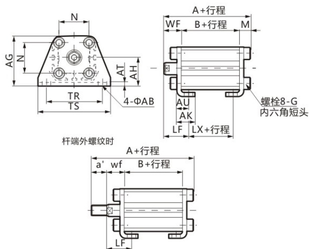
轴向脚座(LB)带开关 SSD2-L-12~25-LB
