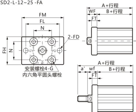
前端法兰(FA)带开关 SSD2-L-12~25-FA
